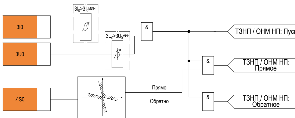
Рисунок 2.29 – Функциональная схема «ОНМ НП»
