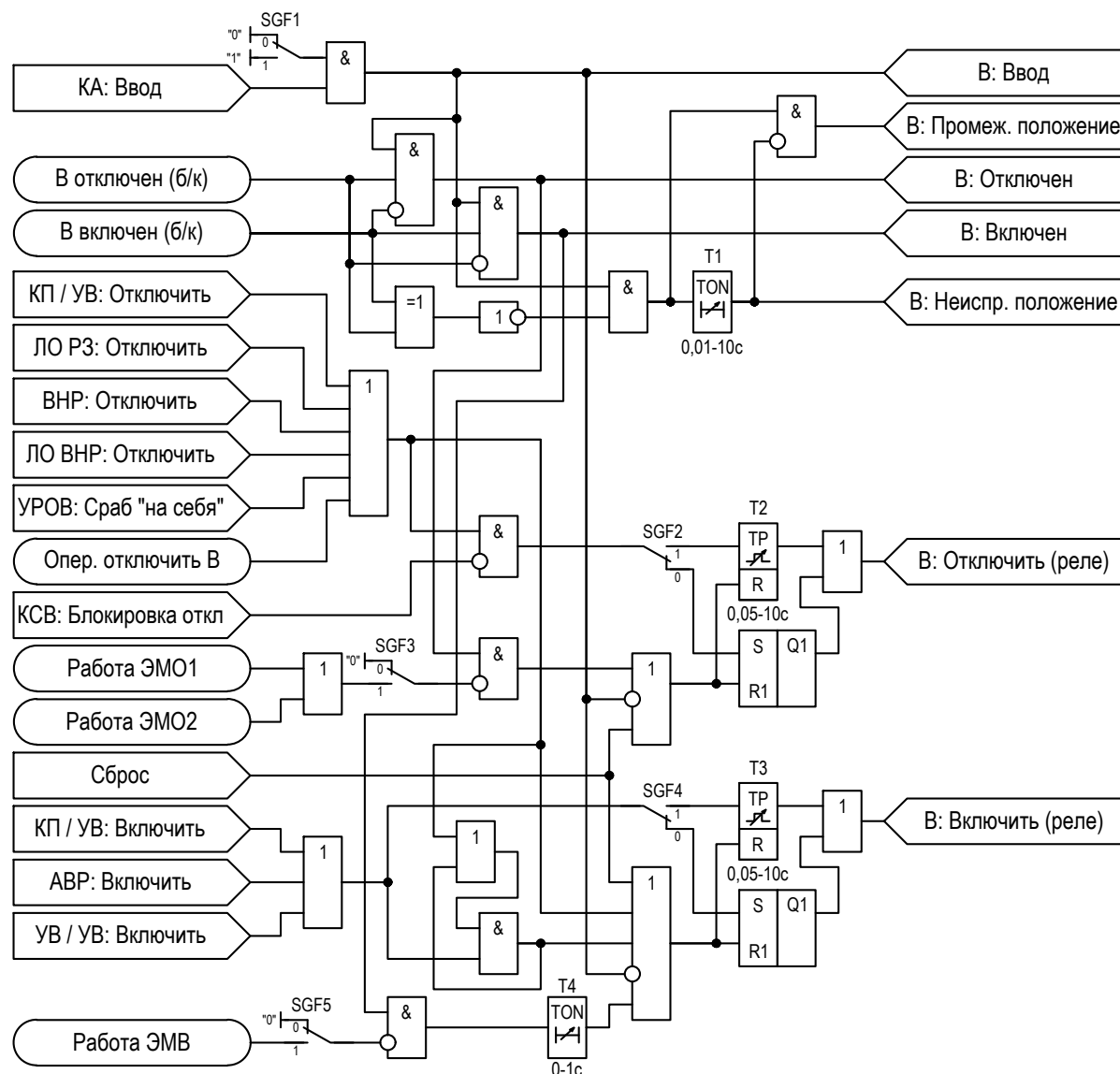
Рисунок 2.57 – Функциональная схема «Выключатель»
