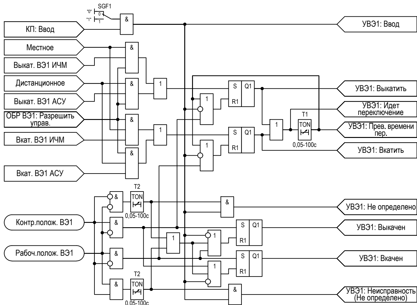
Рисунок 2.49 – Функциональная схема «УВЭ1»
