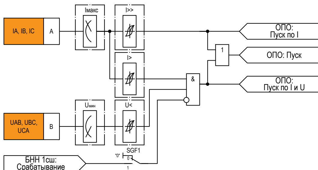
Рисунок 2.7 – Функциональная схема «ОПО ДЗ»
