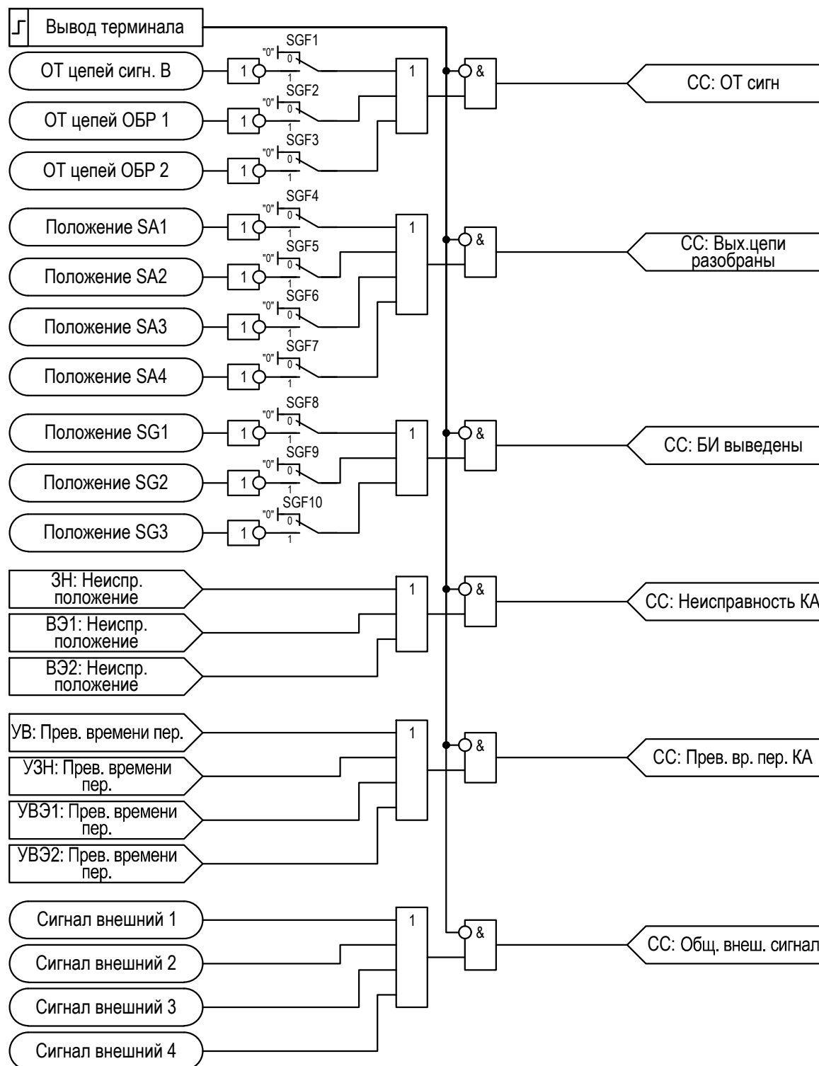
Рисунок 2.62 – Функциональная схема «СС»
