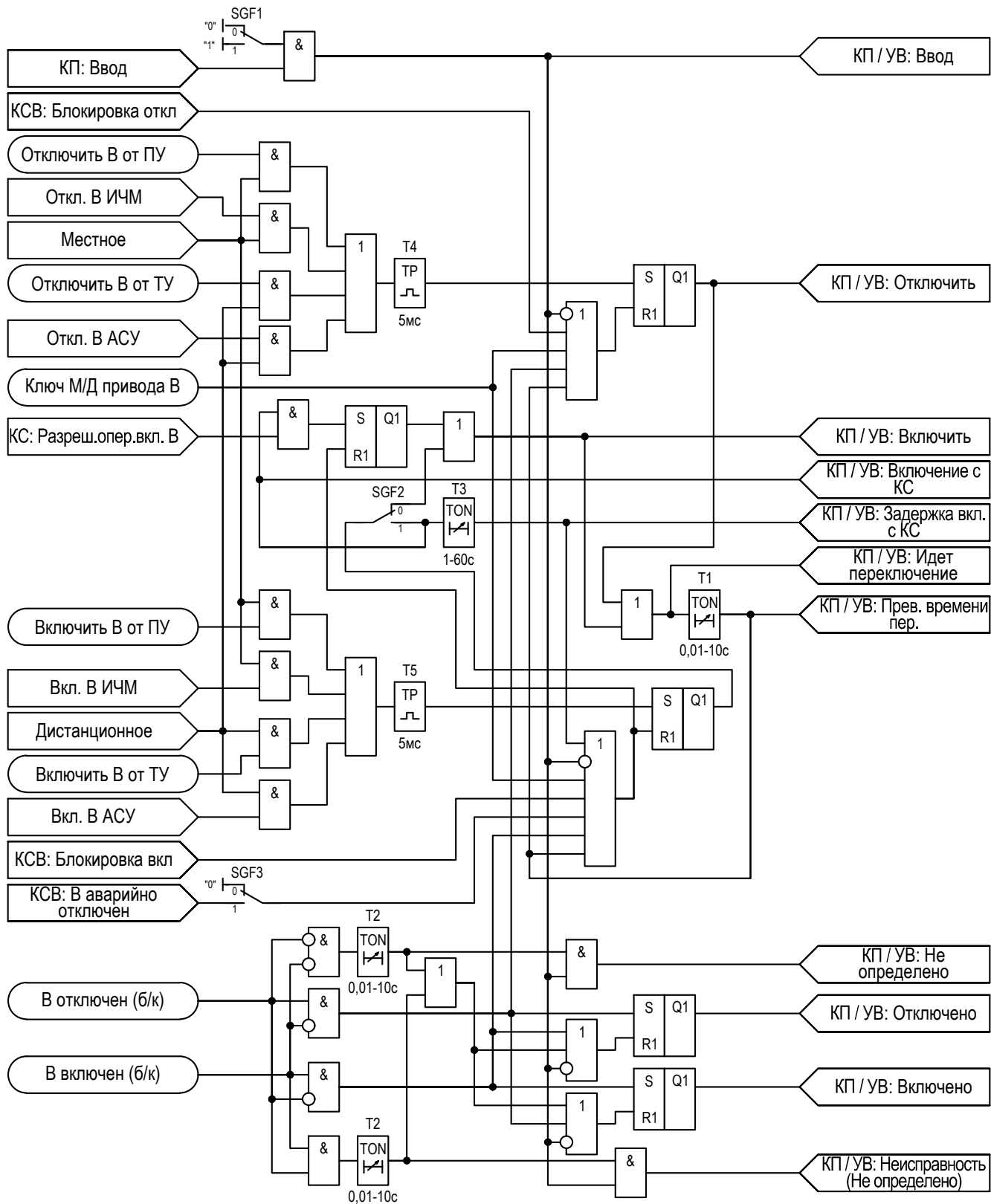
Рисунок 2.47 – Функциональная схема «УВ»
