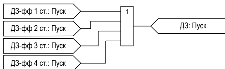
Рисунок 2.10 – Функциональная схема внешней логики ДЗ
