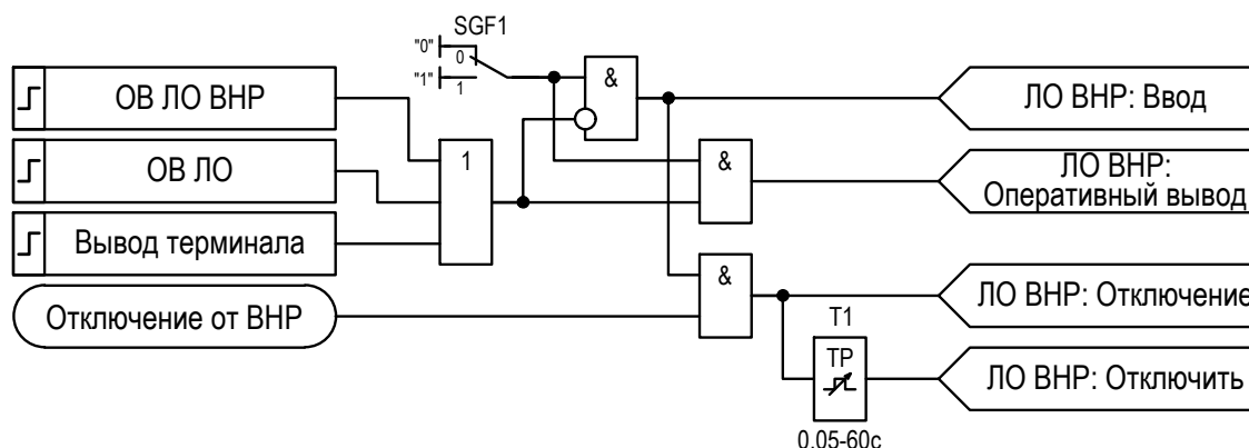
Рисунок 2.43 – Функциональная схема «ЛО ВНР»
