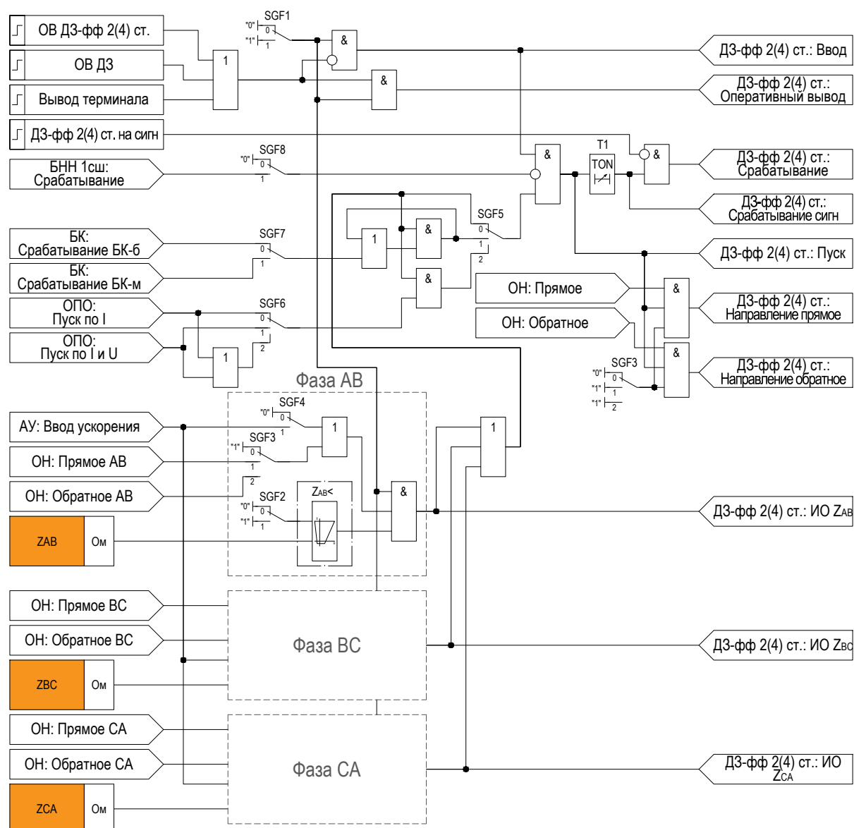
Рисунок 2.3 – Функциональная схема «ДЗ-фф 2(4)ст.»
