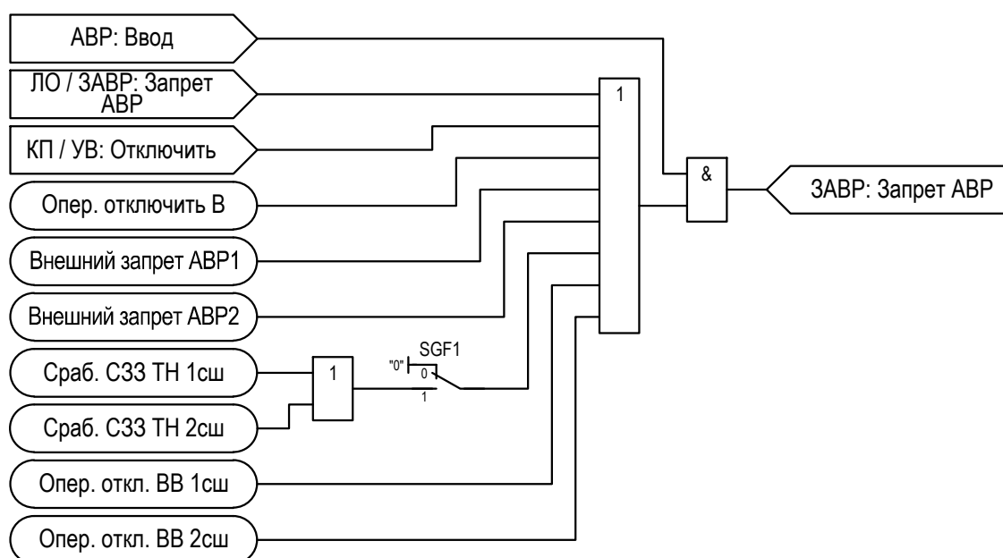
Рисунок 2.40 – Функциональная схема «ЗАВР»
