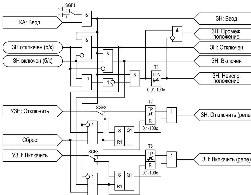
Рисунок 2.58 – Функциональная схема «ЗН»
