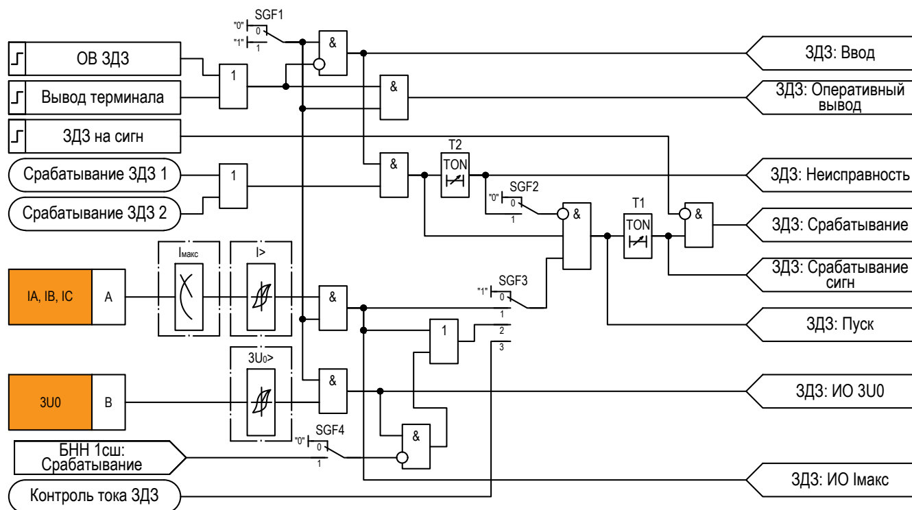
Рисунок 2.24 – Функциональная схема «ЗДЗ»
