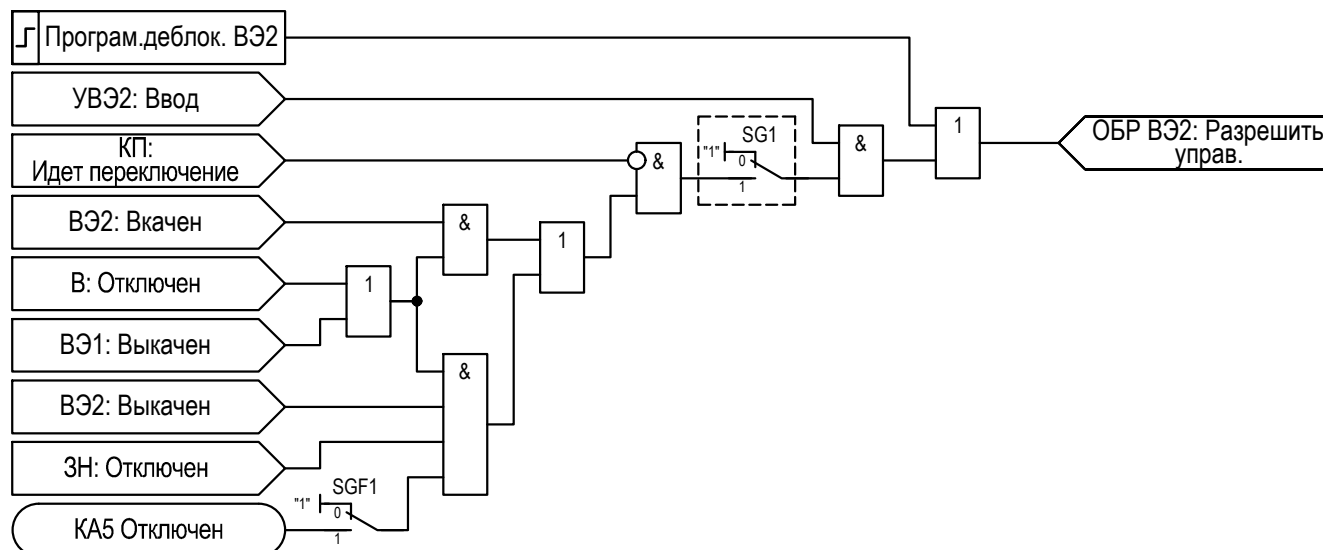
Рисунок 2.54 – Функциональная схема «ОБР ВЭ2»
