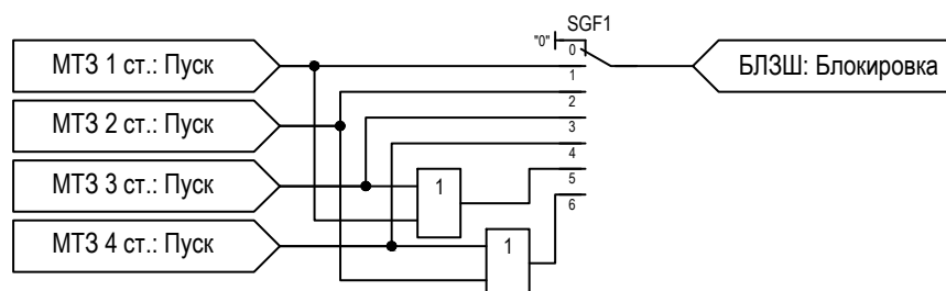
Рисунок 2.19 – Функциональная схема БЛЗШ
