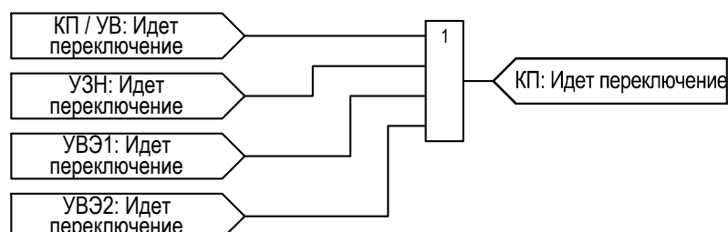
Рисунок 2.46 – Функциональная схема формирования общего сигнала переключения коммутационного аппарата
