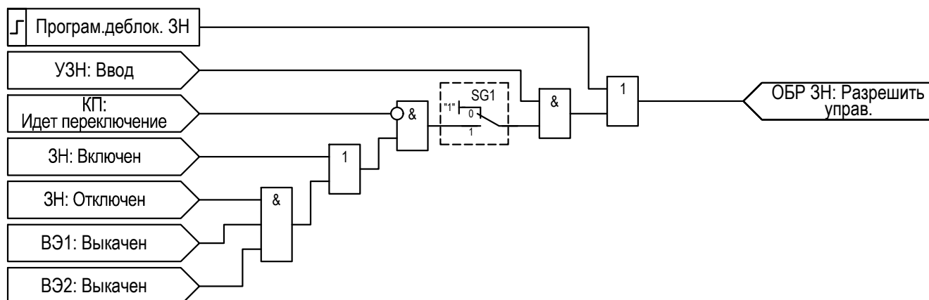
Рисунок 2.52 – Функциональная схема «ОБР ЗН»
