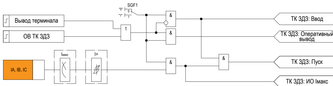
Рисунок 2.25 – Функциональная схема «ТК ЗД3»
