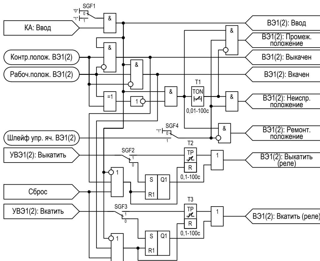
Рисунок 2.59 – Функциональная схема «ВЭ1(2)»
