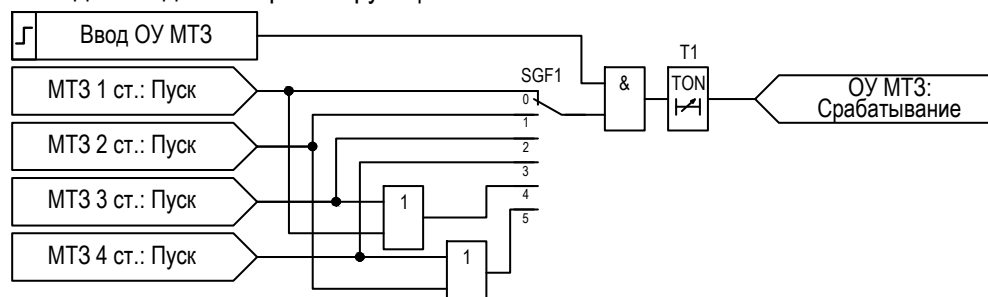
Рисунок 2.21 – Функциональная схема ОУ МТЗ
