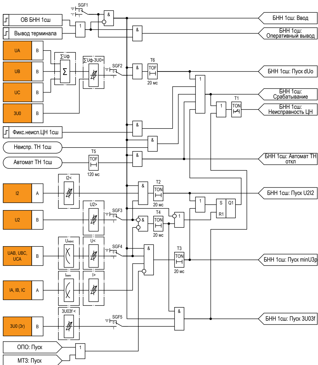
Рисунок 2.34 – Функциональная схема «БНН 1сш»
