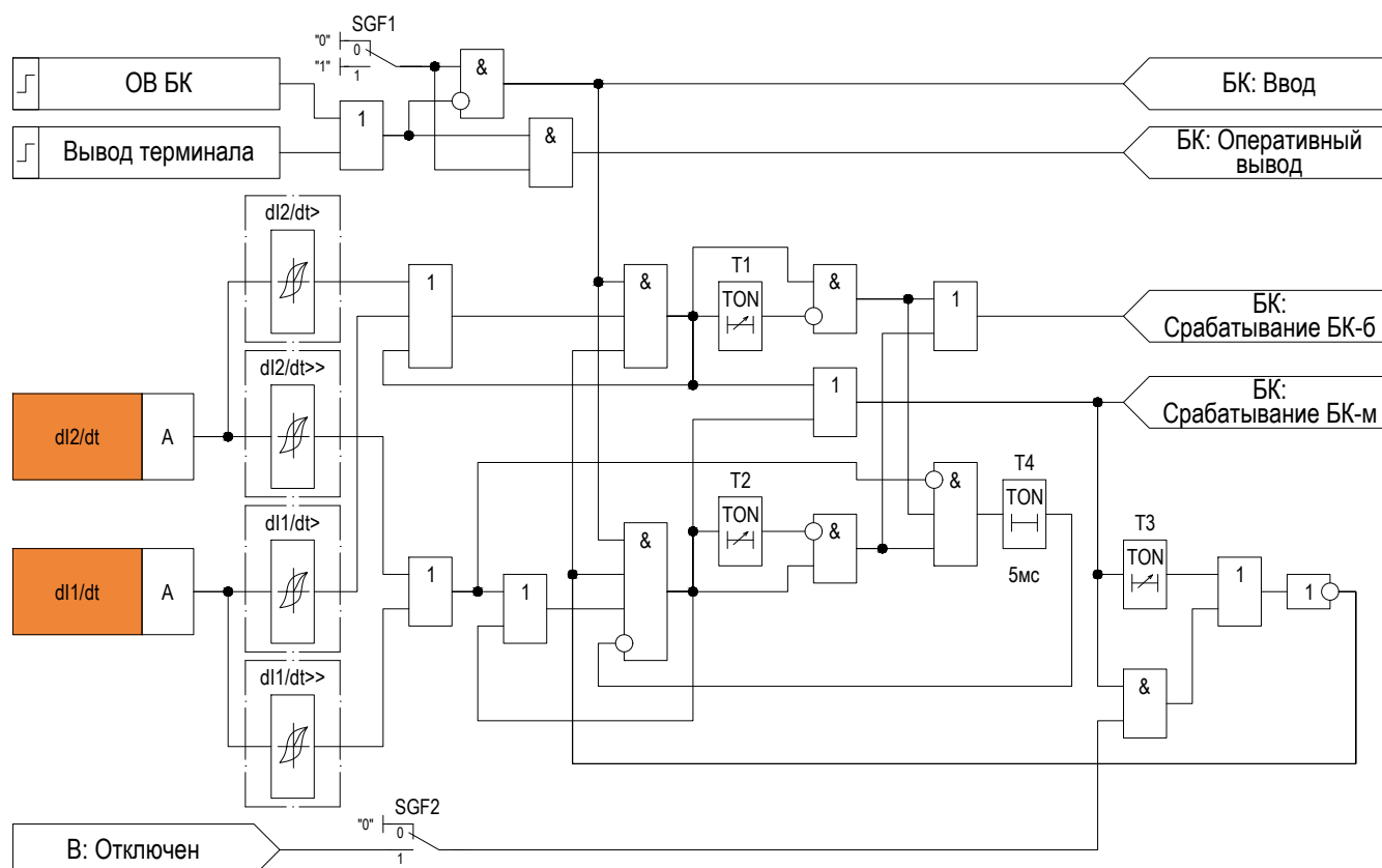
Рисунок 2.11 – Функциональная схема «БК»
