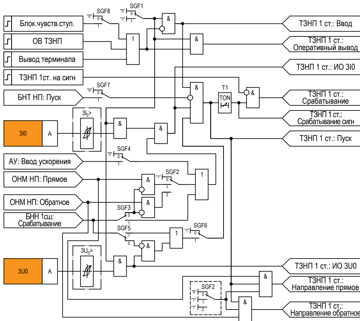
Рисунок 2.27 – Функциональная схема ступеней ТЗНП
