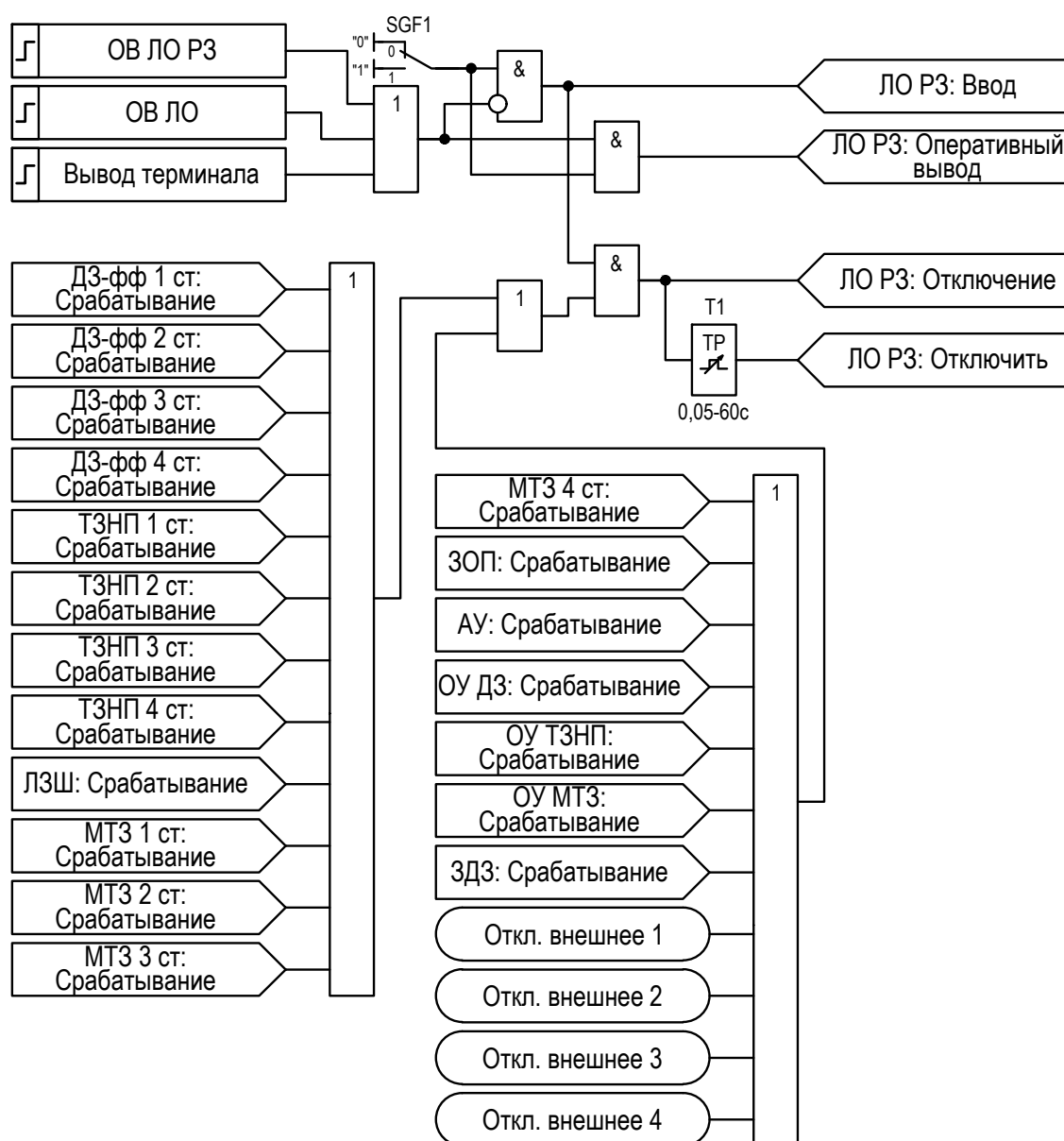
Рисунок 2.42 – Функциональная схема «ЛО РЗ»
