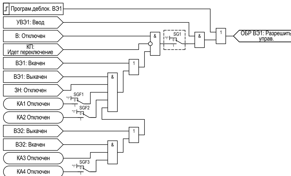
Рисунок 2.53 – Функциональная схема «ОБР ВЭ1»
