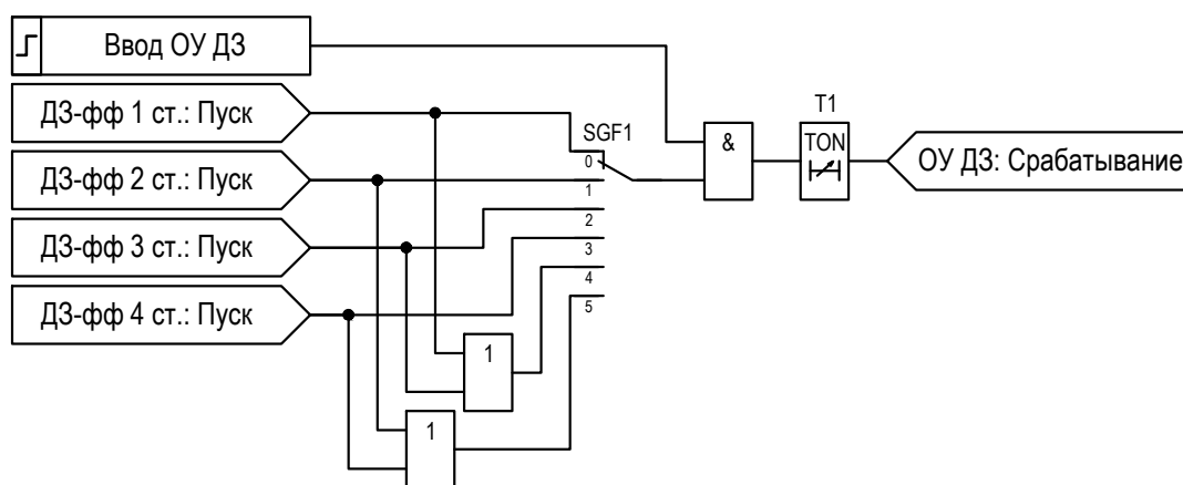
Рисунок 2.9 – Функциональная схема «ОУ ДЗ»
