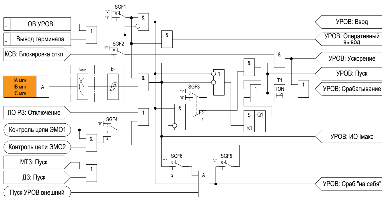
Рисунок 2.33 – Функциональная схема «УРОВ»
