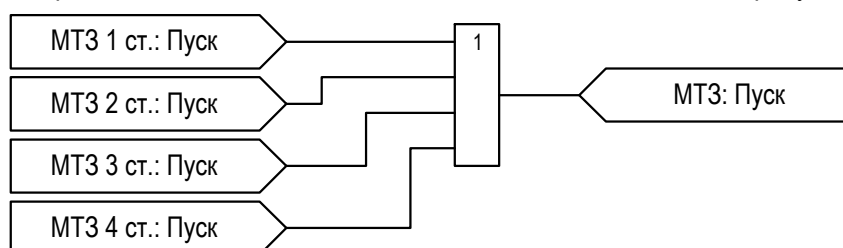
Рисунок 2.22 – Функциональная схема внешней логики МТЗ
