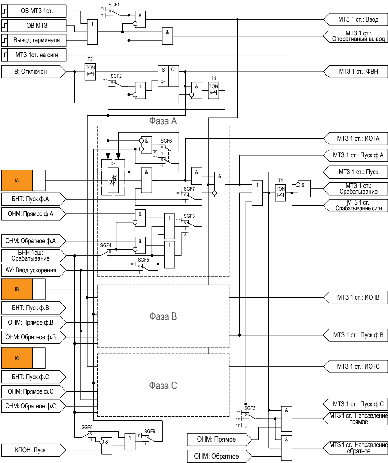
Рисунок 2.13 – Функциональная схема ступени МТ3
