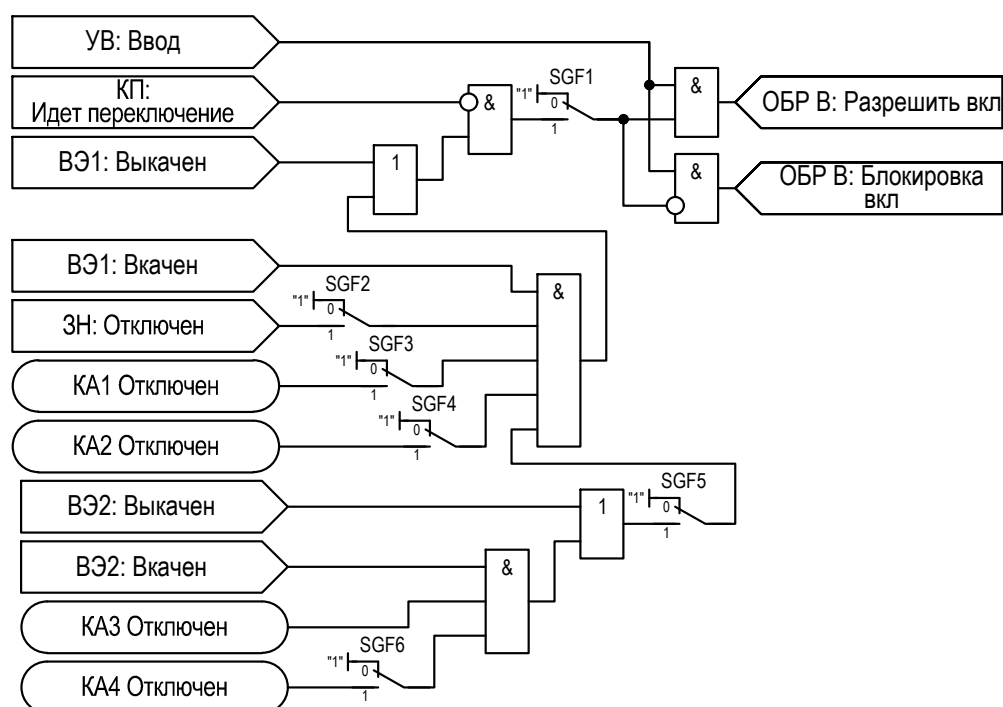
Рисунок 2.51 – Функциональная схема «ОБР В»
