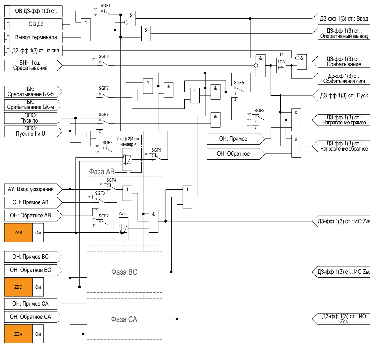
Рисунок 2.2 – Функциональная схема «ДЗ-фф 1(3)ст.»
