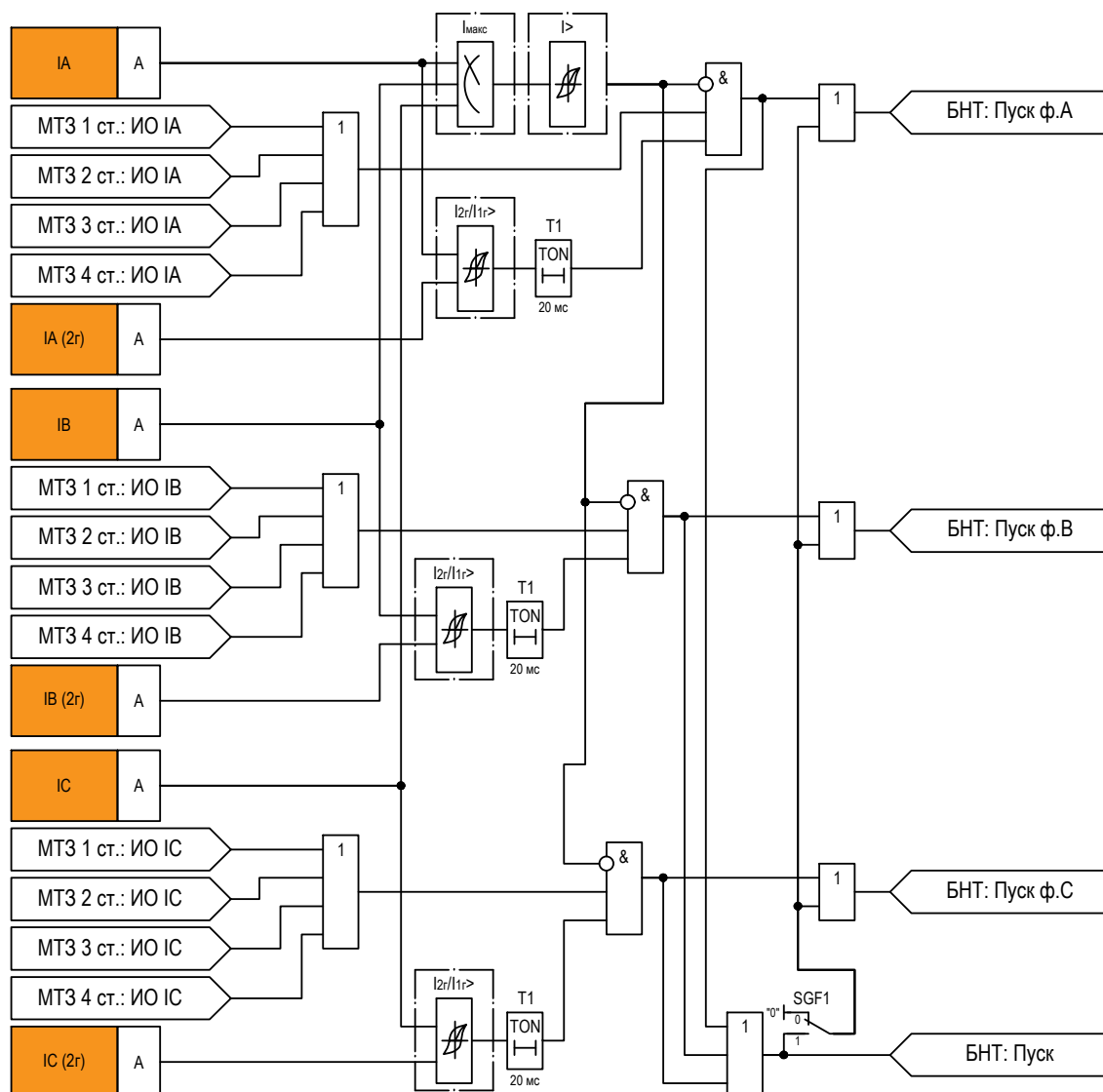
Рисунок 2.18 – Функциональная схема «БНТ»
