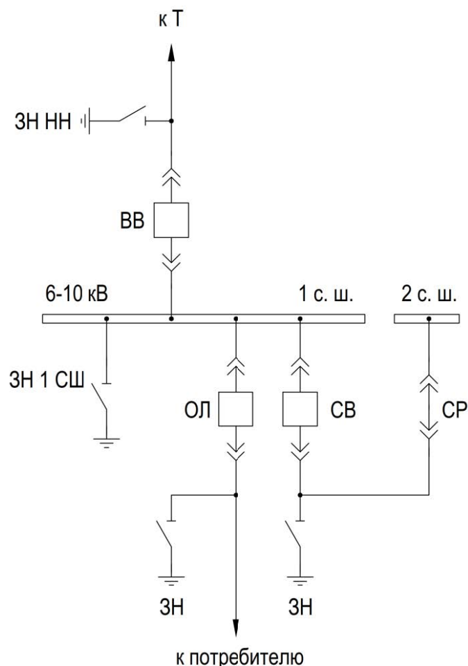
Рисунок 2.50 – Поясняющая схема первичной сети для алгоритмов оперативной блокировки КА
