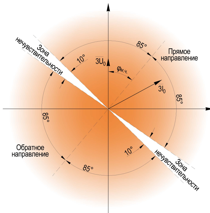
Рисунок 2.28 – Характеристика органа направления мощности нулевой последовательности
