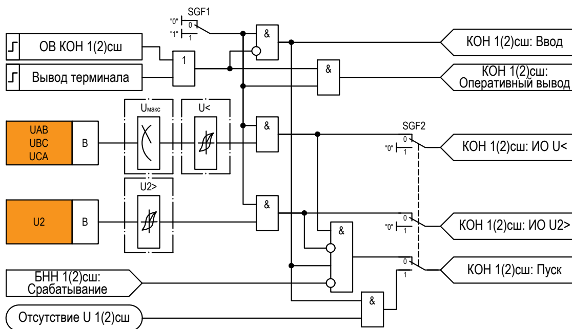
Рисунок 2.37 – Функциональная схема «КОН 1(2)сш»
