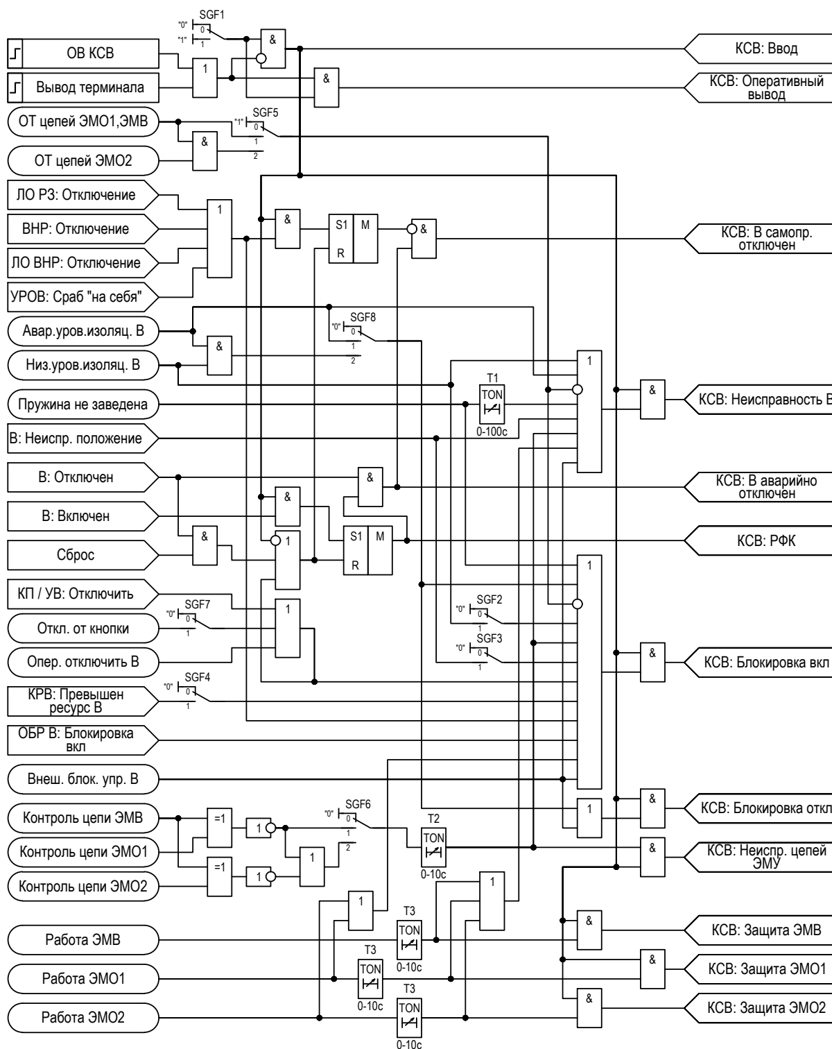
Рисунок 2.60 – Функциональная схема «КСВ»
