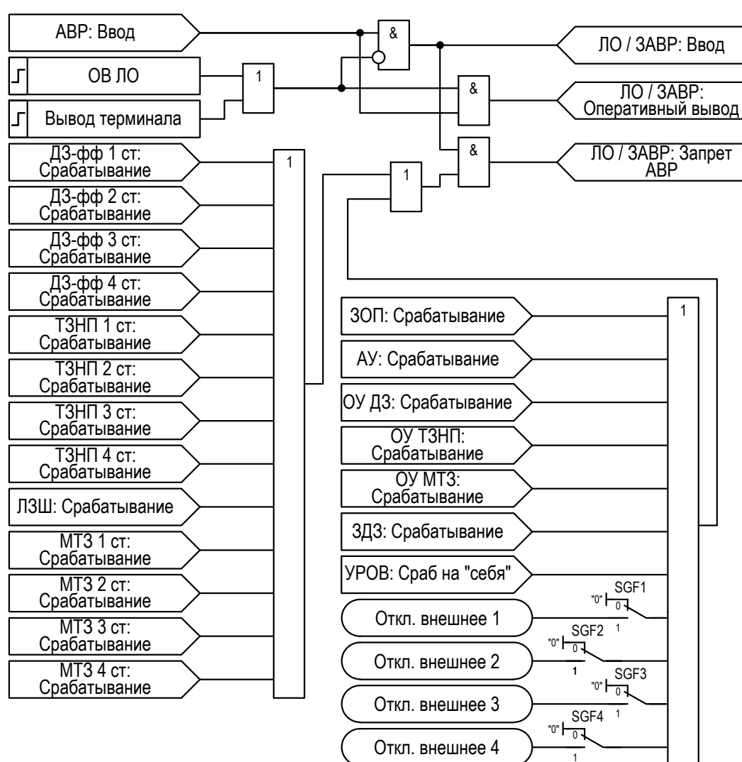
Рисунок 2.44 – Функциональная схема «ЗАВР ЛО»
