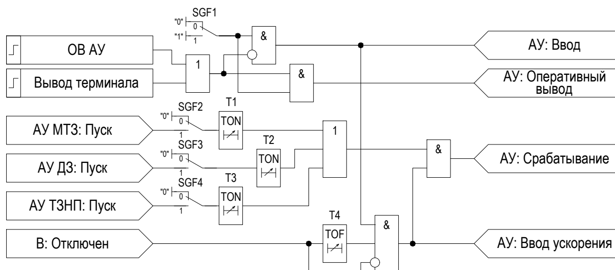
Рисунок 2.12 – Функциональная схема «АУ»
